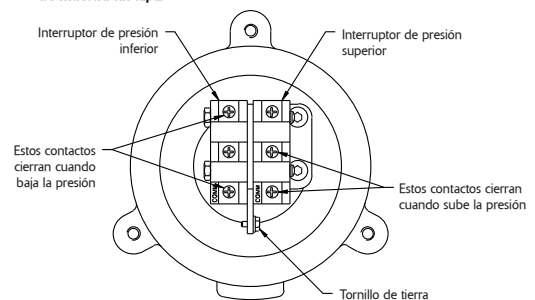
Vista superior (se muestra sin tapa)
